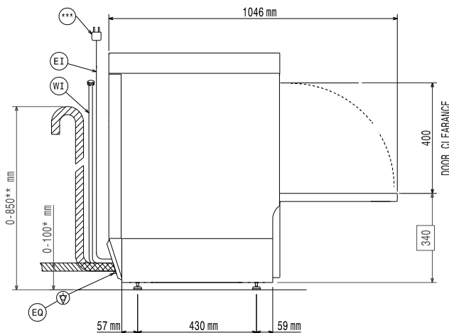
Zij aanzicht
